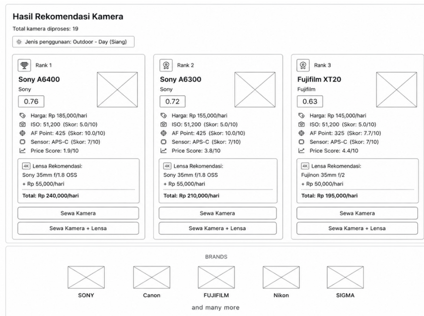
Gambar 4. 18 Hasil Rekomendasi Kamera
