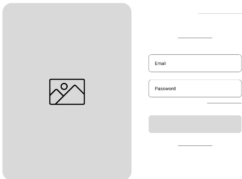
Gambar 4. 9 Wireframe Login
