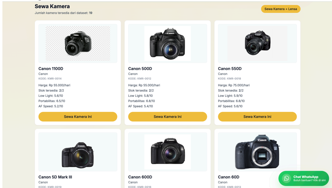
Gambar 4. 28 Katalog Kamera
